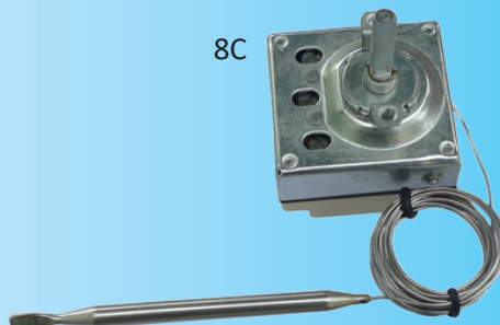
3-полюсный патронный и капиллярный термостат, диапазон температур до 320°C
